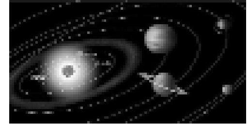
Gökyüzünde sadece güneş sistemindeki değil, evrendeki tüm gök cisimlerinin bir yörüngesi vardır.
