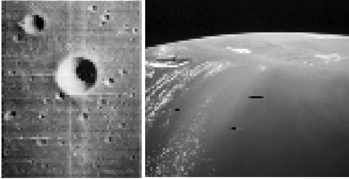
Ay'ın Dünya gibi koruyucu bir atmosferi olmadığı için sürekli göktaşı bombardımanı altındadır. Ay'ın yüzeyi göktaşlarının darbeleriyle kraterlerle doludur.
