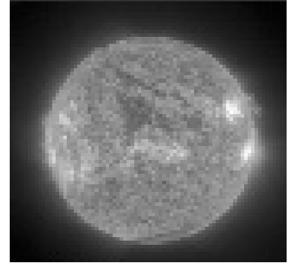
Meton devrinde güneş kendi eksenini etrafında tam 475 sefer döner.
