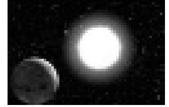
Güneş, güneş sisteminin merkezinde olmasına rağmen kendisine ait bir yörüngede evren içinde hareket etmektedir.
