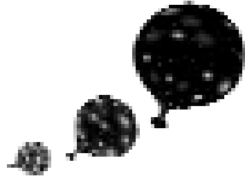
Evren şişen bir balon gibi sürekli genişlemekte ve gök yüzündeki tüm cisimler birbirinden uzaklaşmaktadır.
